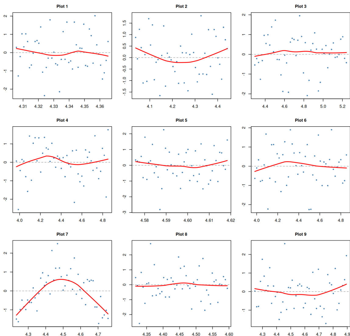
Hình 10: Giao thức xếp hàng: 8 đồ thị nền và 1 đồ thị phần dư thực (mô hình bậc 1 trên dữ liệu cong). Xác suất đoán ngẫu nhiên đúng là 1/9 \approx 11\% . Nếu bạn nhận ra đồ thị thực, đó là bằng chứng thị giác có ý nghĩa thống kê. Hữu ích nhất khi n < 30 và mẫu hình phần dư mơ hồ. (Đáp án: Đồ thị 7.)
